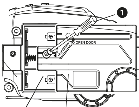
Paristojen asettaminen
