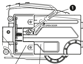
Batterij Installatie
